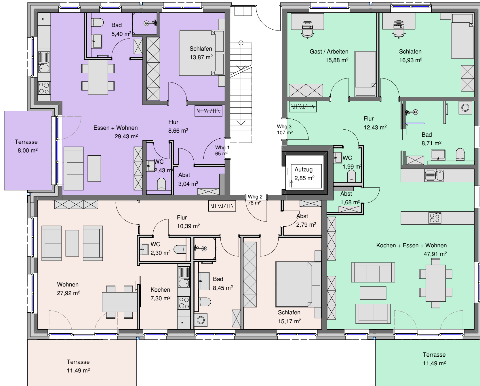
Grundriss Erdgeschoss
